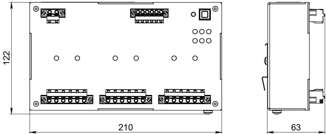
Рисунок Б.1 – Габаритные размеры HCR-06F Ex
