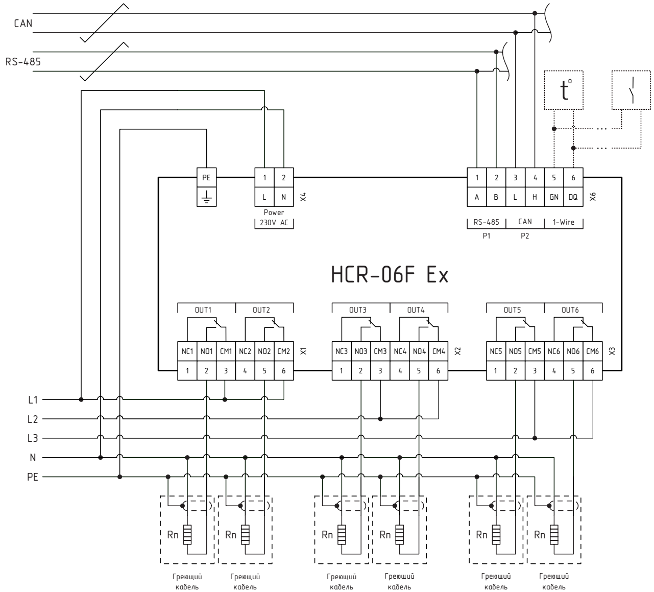
Рисунок В.2 – Схема подключения HCR-06F Ex
