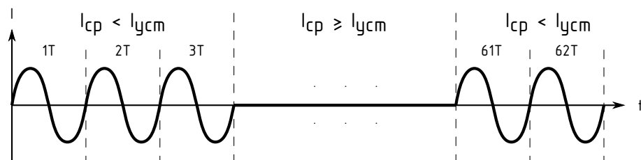
Рисунок 2.7 – Режим «Ограничение тока»
