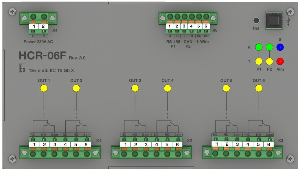
Рисунок 2.1 – Внешний вид устройства HCR-06F Ex
