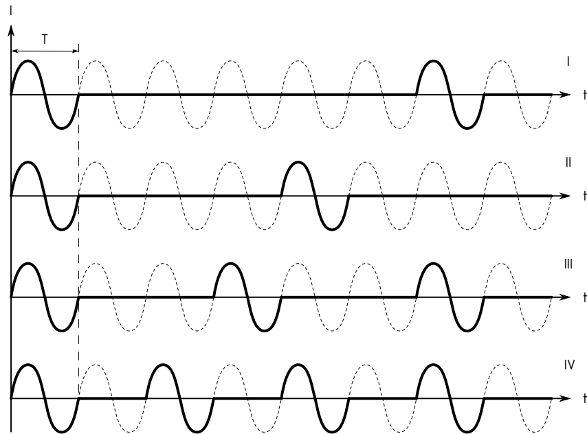
Рисунок 2.6 – Режим «Плавный пуск»
